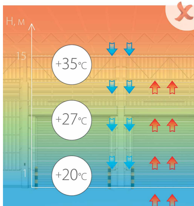
Распределение тепла в здании без использования дестратификаторов
